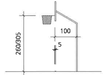
Mst. 1:100
