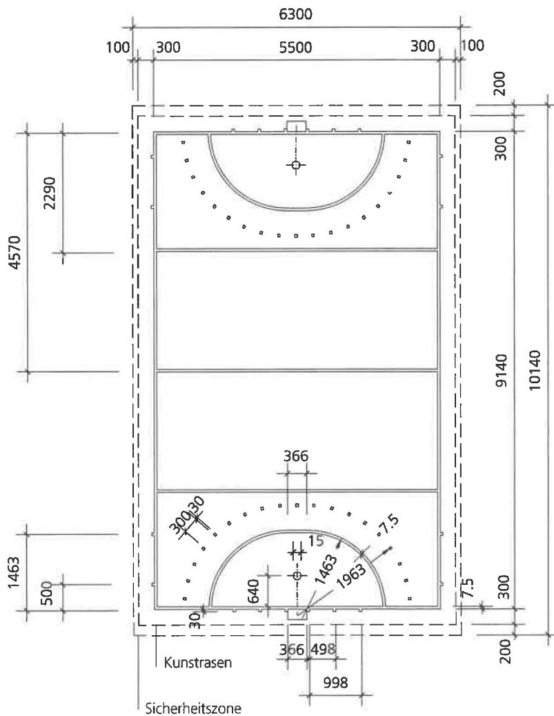
Mst. 1:1000
