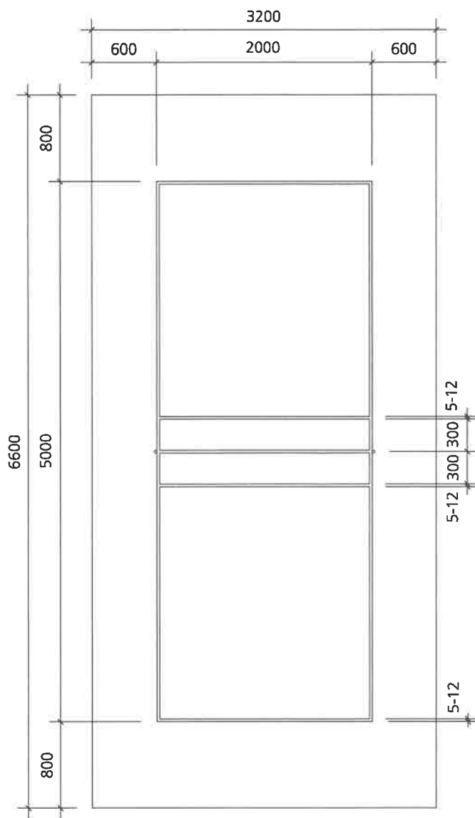
Mst. 1:500
