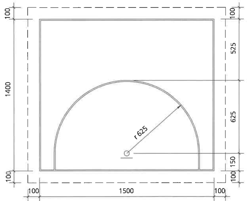
Mst. 1:200
