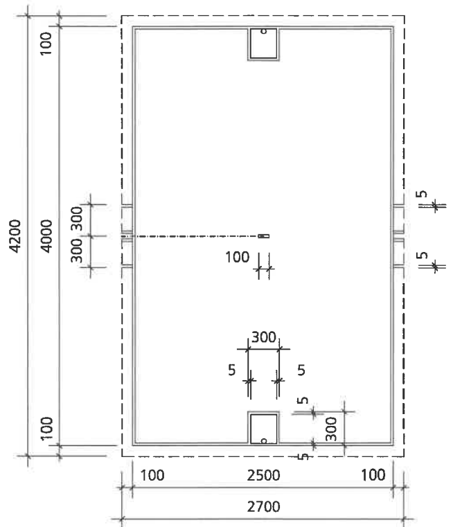
Mst. 1:500
